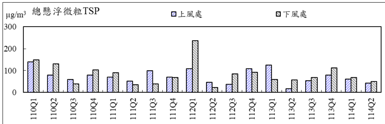
圖 2.1- 1 空氣品質總懸浮微粒(24 小時值)監測結果
