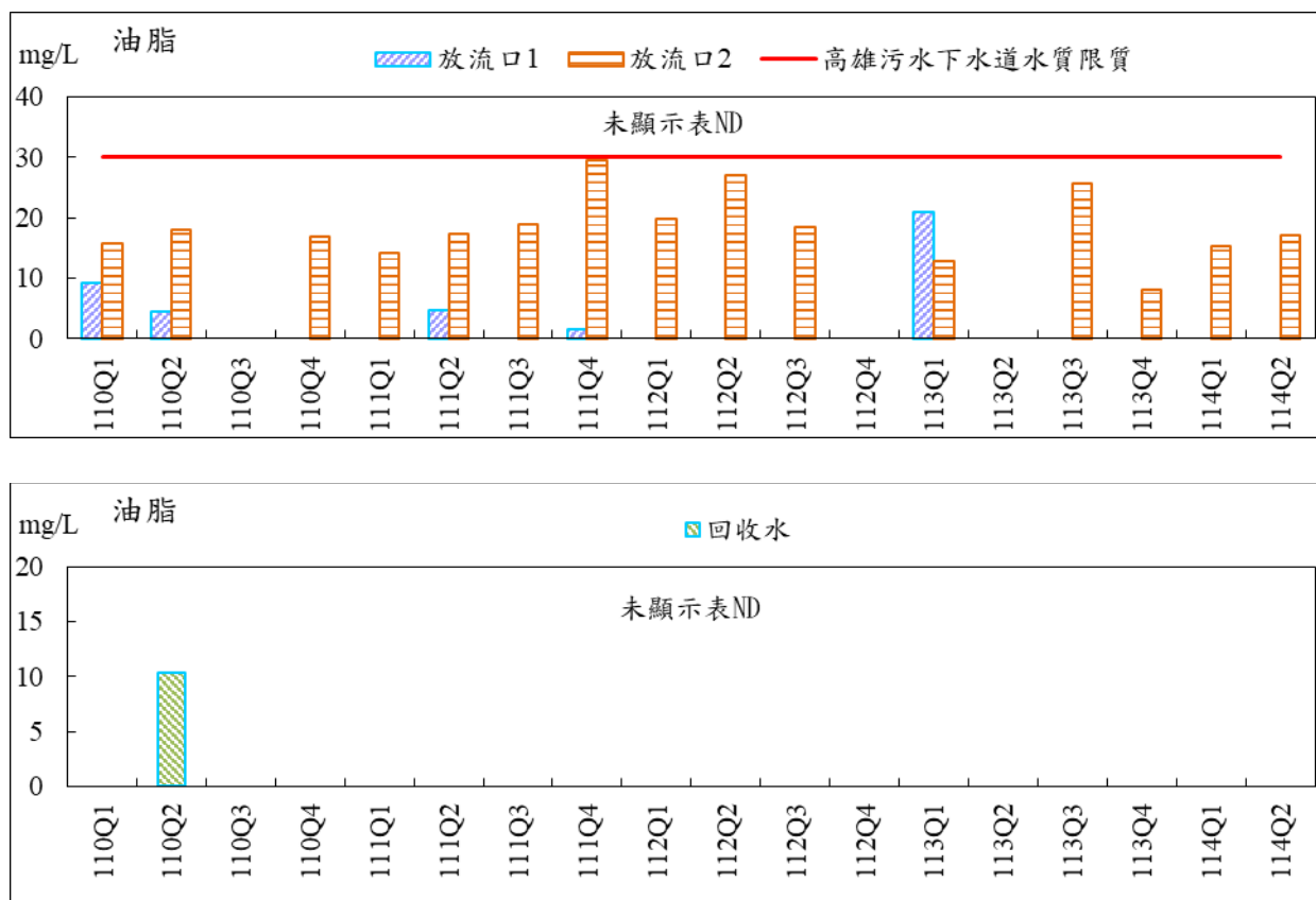
圖 2.3- 7 水質油脂監測結果
