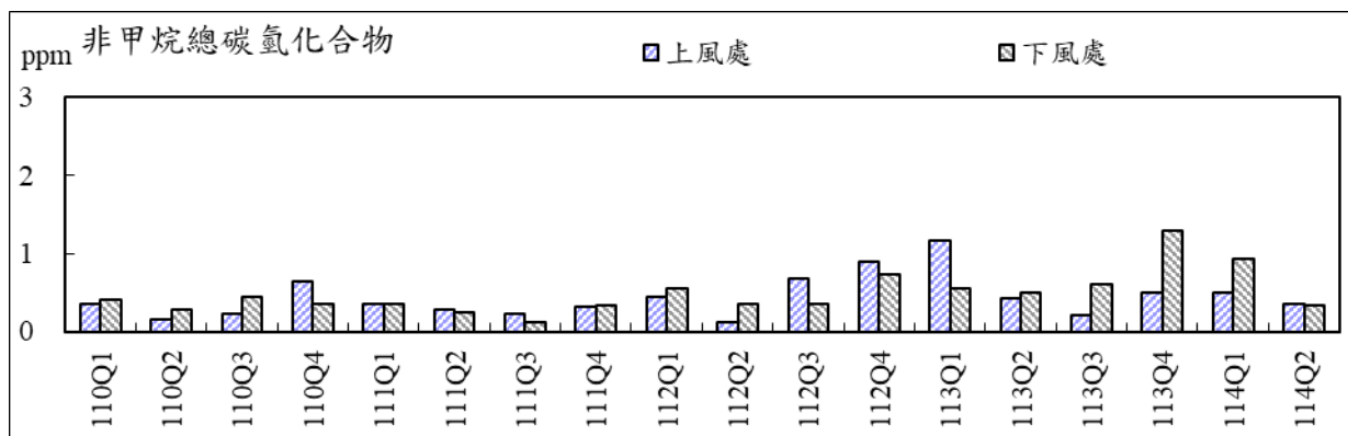
圖 2.1- 12 空氣品質非甲烷總碳氫化合物(小時平均值)監測結果
