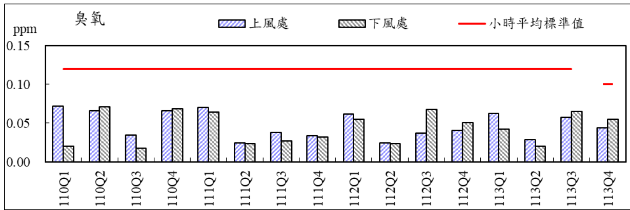
圖 2.1- 9 空氣品質臭氧(小時平均值)監測結果
