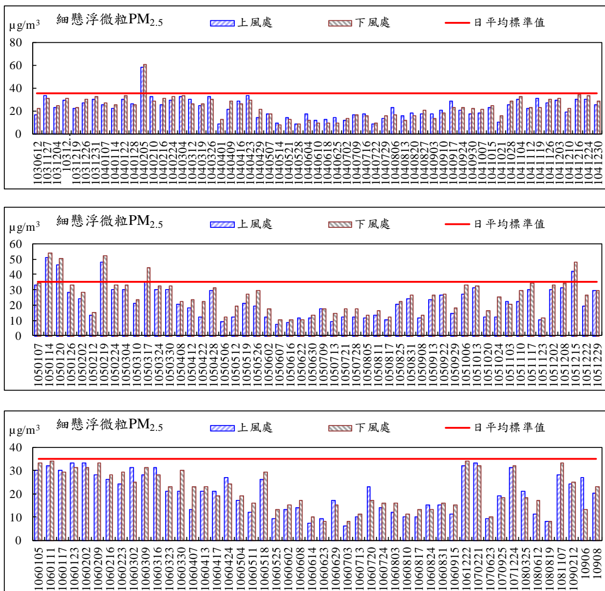
圖 2.1- 13 空氣品質細懸浮微粒(24 小時平均值)監測結果
