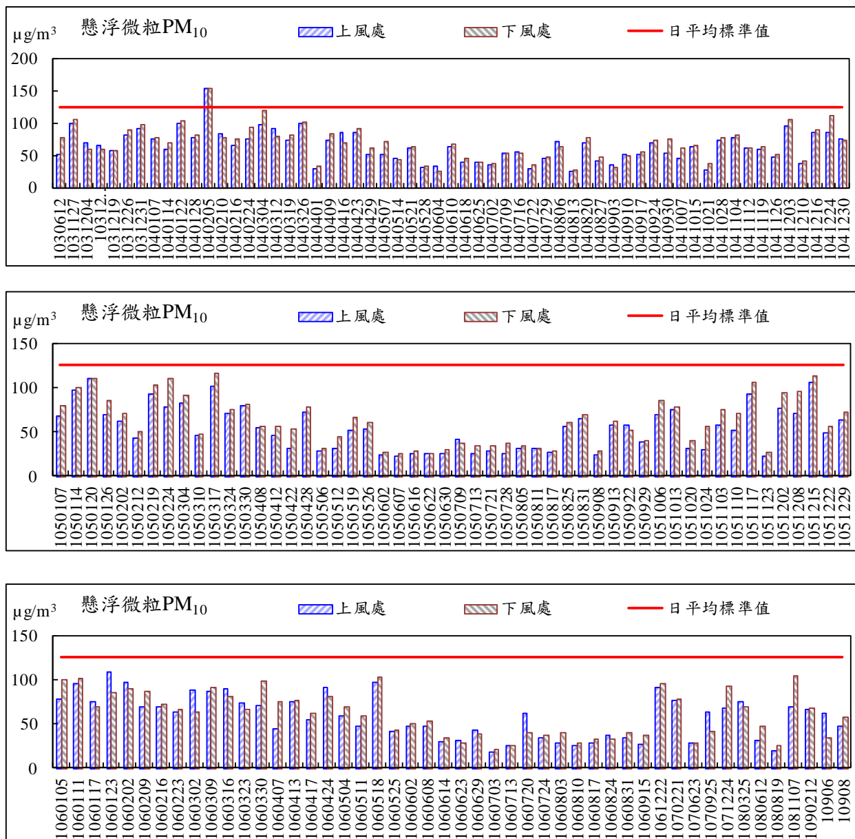
圖 2.1- 12 空氣品質懸浮微粒(日平均值)監測結果
