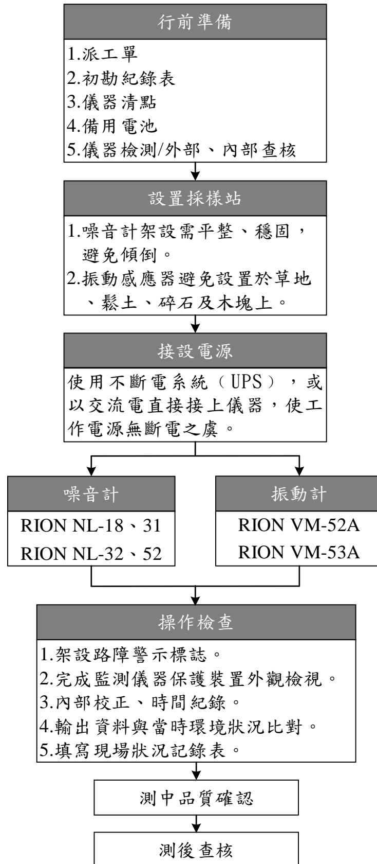
圖 1.5- 2 噪音振動現場採樣流程
