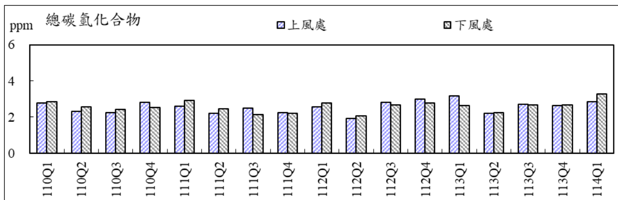
圖 2.1- 11 空氣品質總碳氫化合物(小時平均值)監測結果
