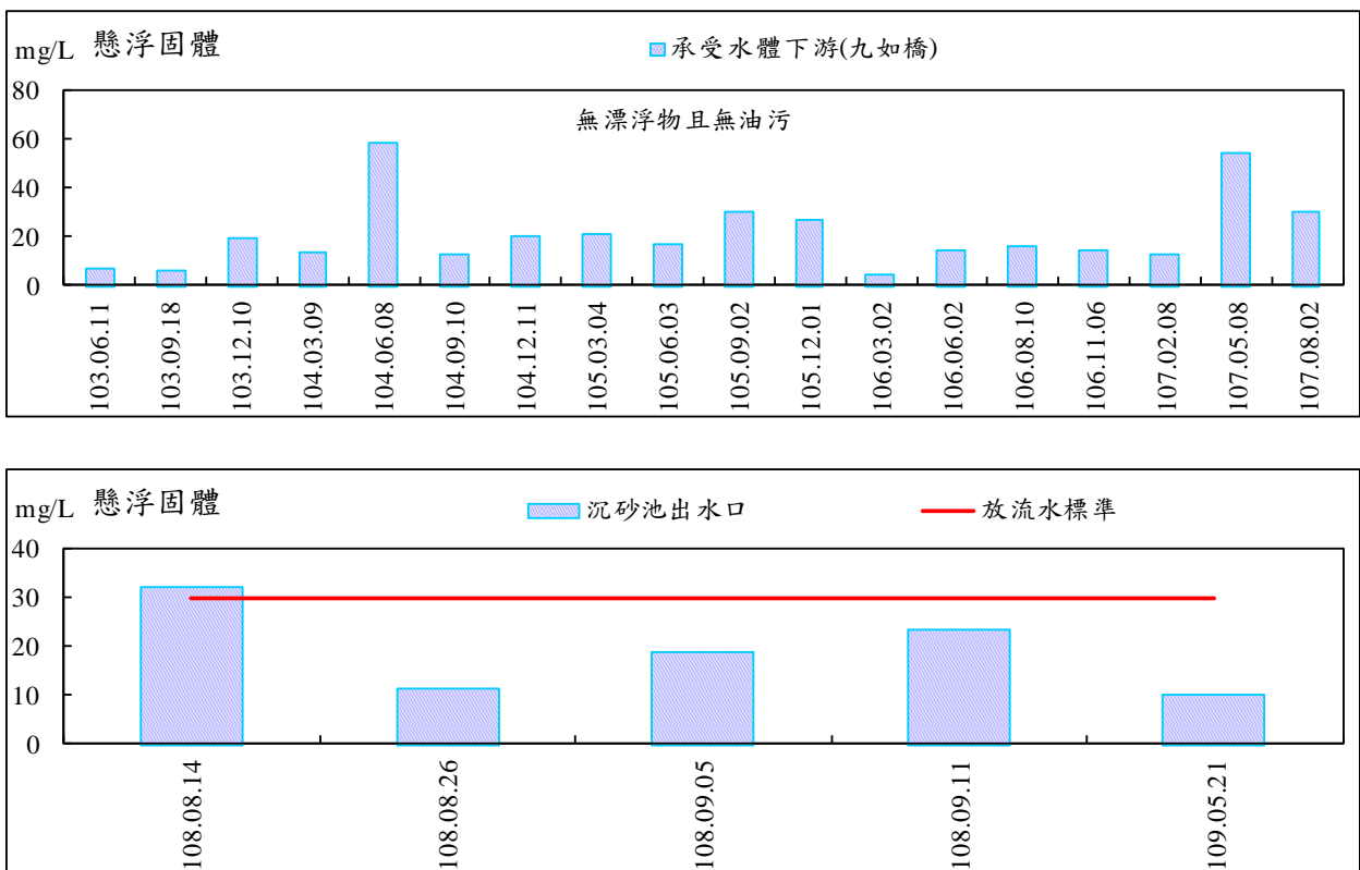
圖 2.3-3 水質懸浮固體監測結果
