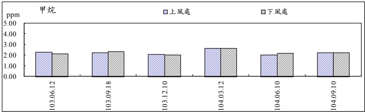
圖 2.1-9 空氣品質甲烷(小時平均值)監測結果
