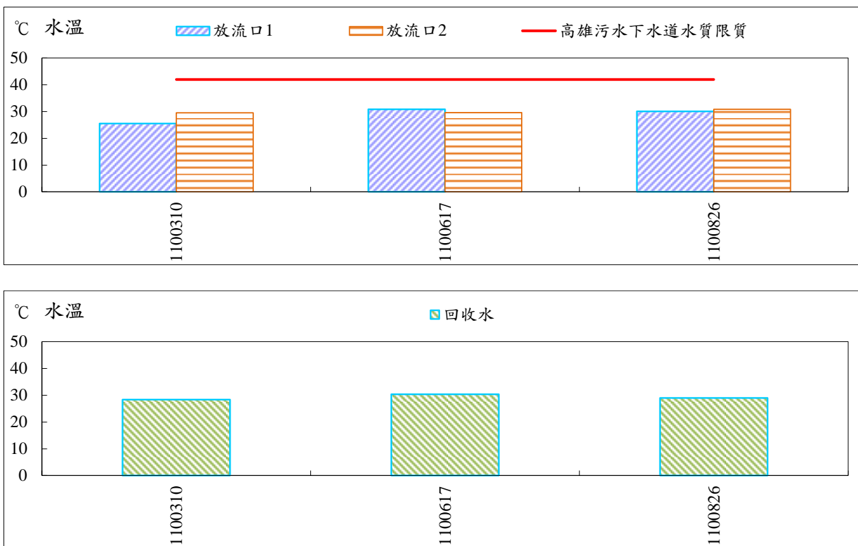
圖 2.3- 2 水質水溫監測結果
