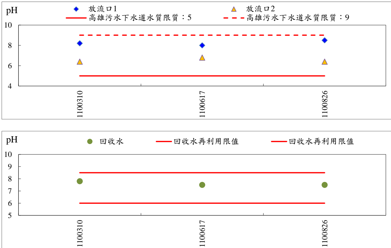
圖 2.3- 1 水質氫離子濃度指數監測結果
